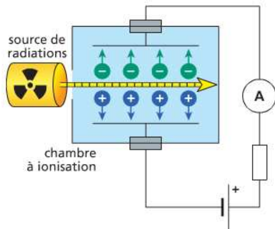
Fig. 1 Modélisation du compteur Geiger-Müller.
